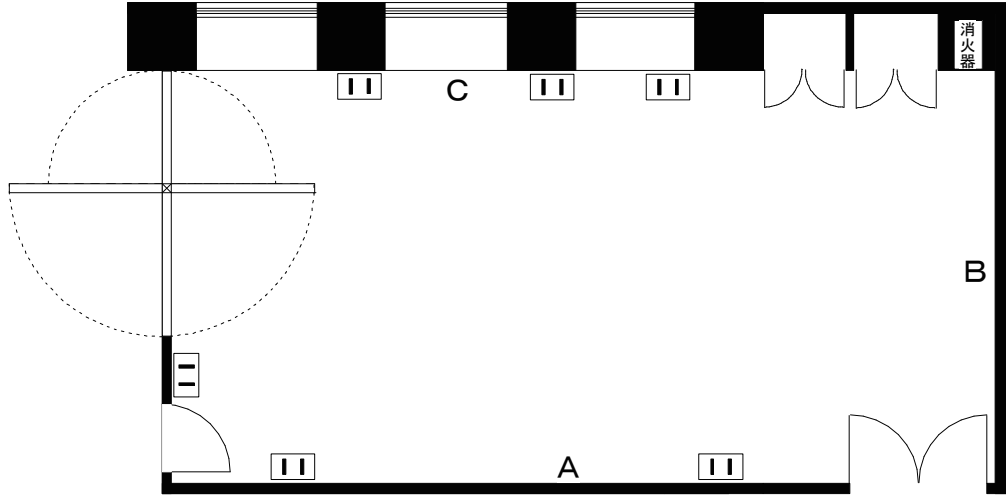
平面図
