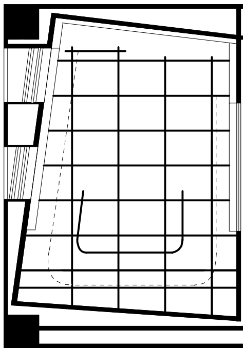
バトン配置図 \phi 45\text{mm}
