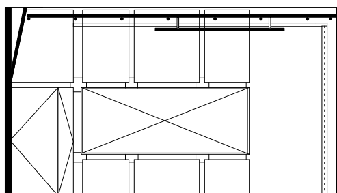
側面図 (仕切窓方向)
